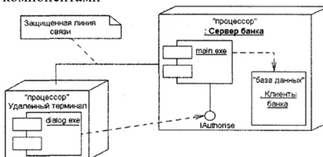
Рисунок 3. Диаграмма развертывания для системы удаленного обслуживания клиентов банка
